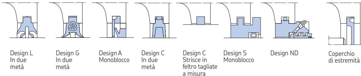
Supporto della serie 2
