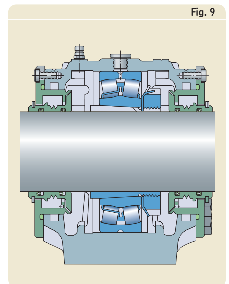
Supporto per la lubrificazione ad olio
