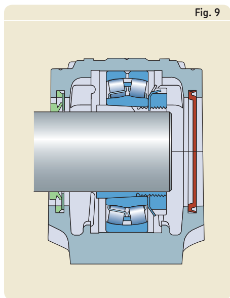
Supporto con coperchio di estremità
