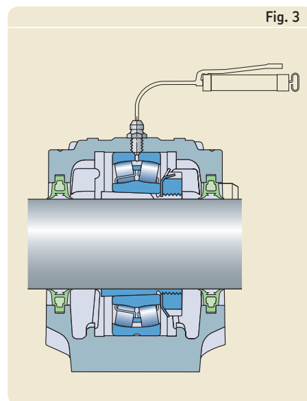
Rilubrificazione del cuscinetto attraverso l'anello esterno (scanalatura W33)
