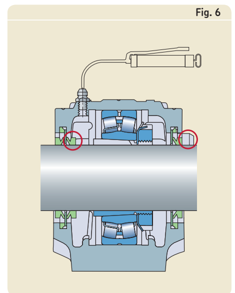
Supporto con V-ring supplementare e piastra paraspruzzi
