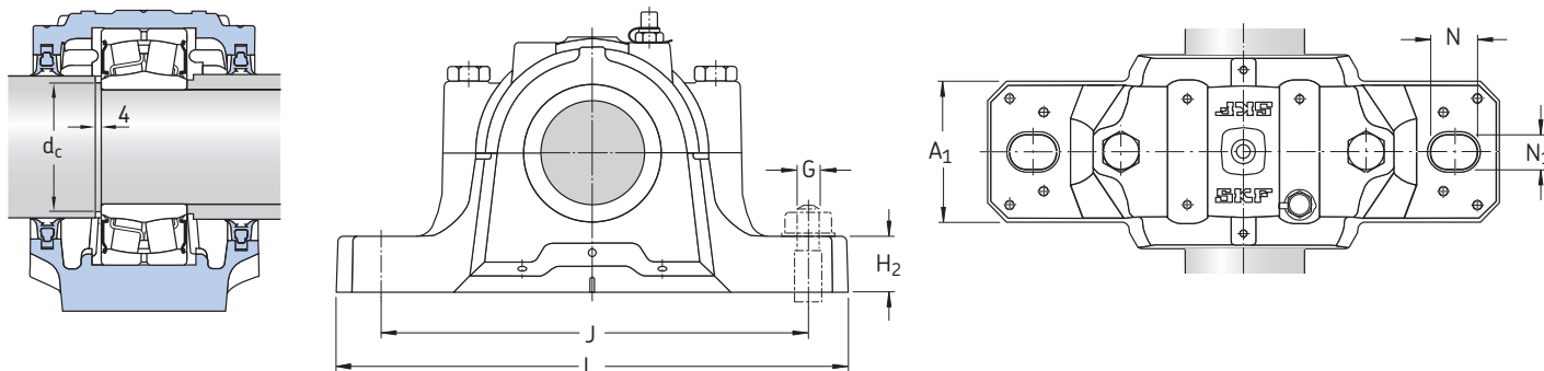
Supporto con cuscinetto orientabile a rulli con tenuta incorporata
