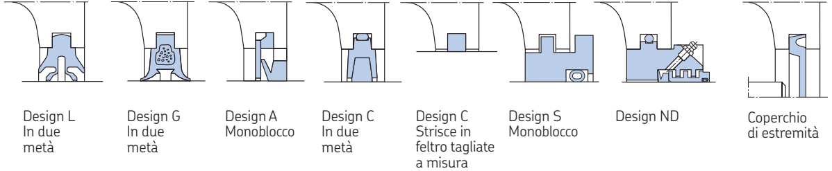
Supporto della serie 2
