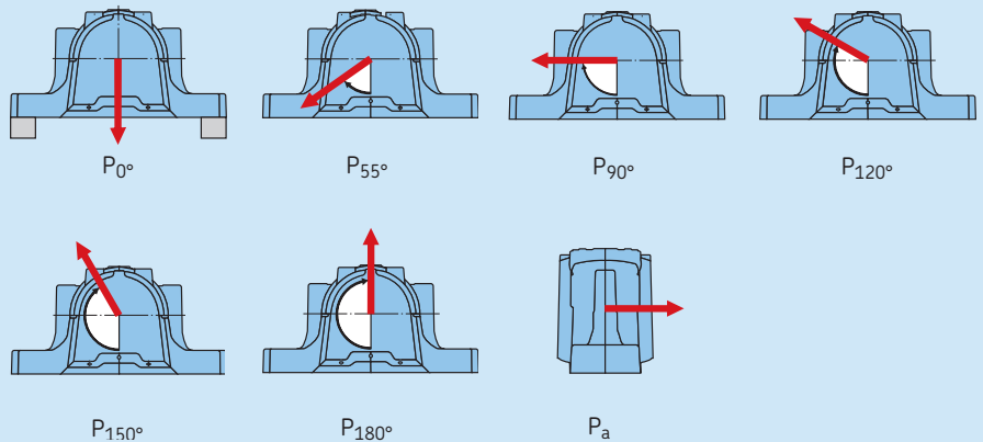
Carichi di rottura per supporti ritzi SNL
