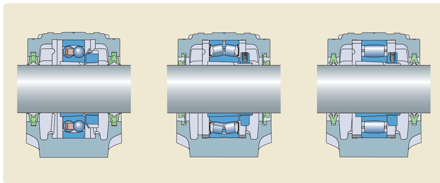
Cuscinetti su bussola di trazione su alberi lisci
