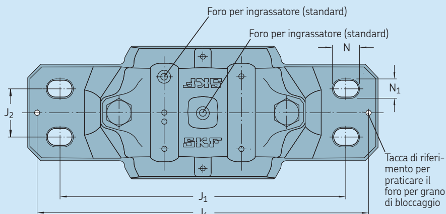
Dimensioni per quattro fori oblungi di fusione per bulloni
